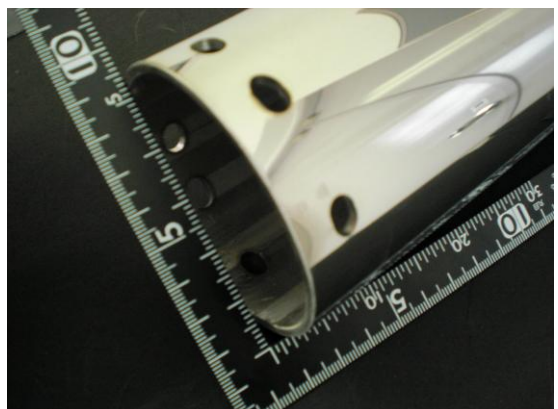
加工例2 SUS304丸パイプ 3.0t クリーンカット
